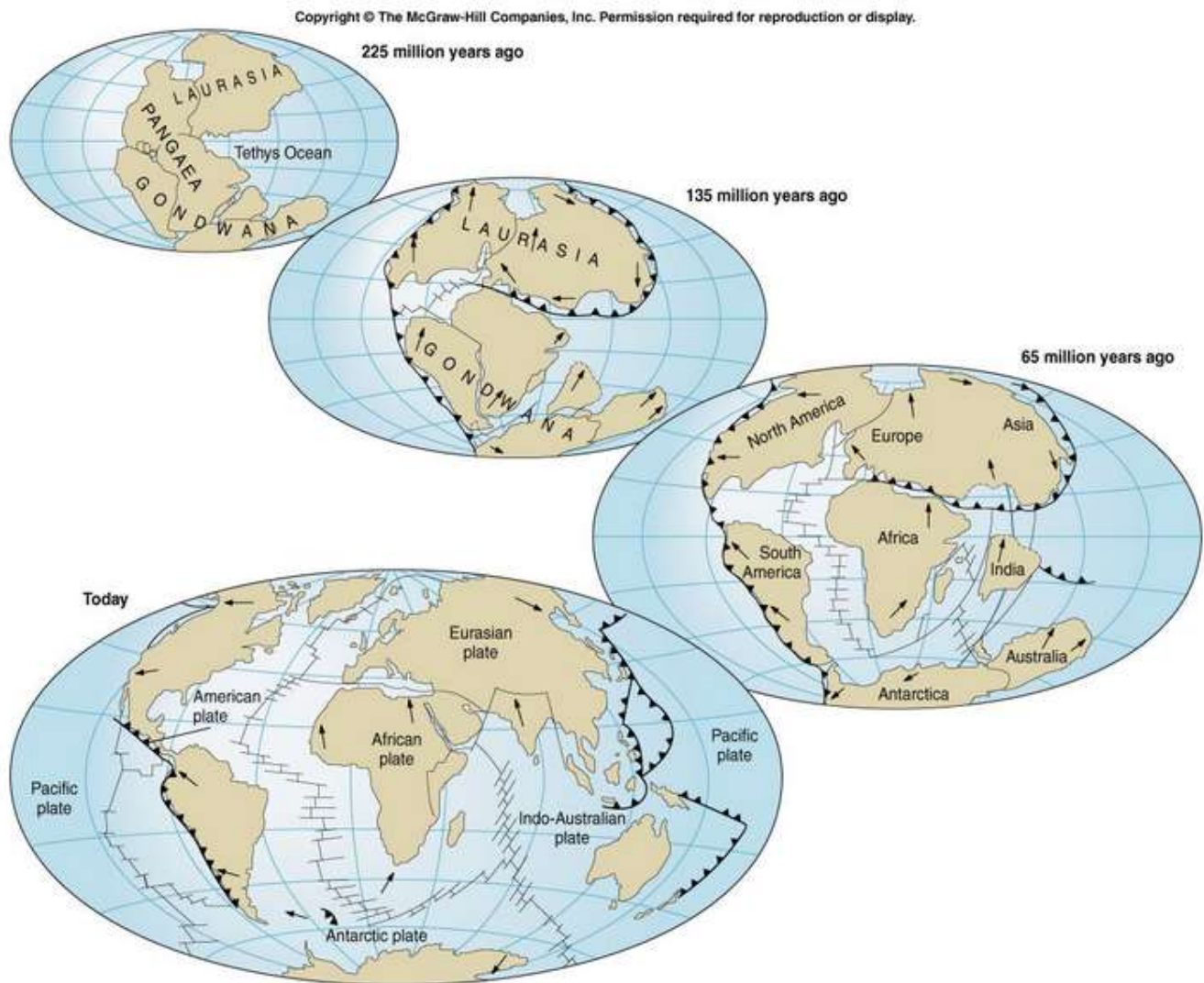
A Pangeia e a sua fragmentação dando origem aos continentes e oceanos que conhecemos hoje.
